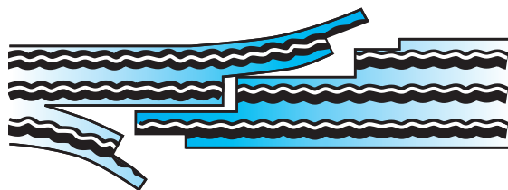
3-lagiger Gurt
