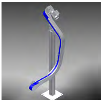
3-D Kettenförderer
